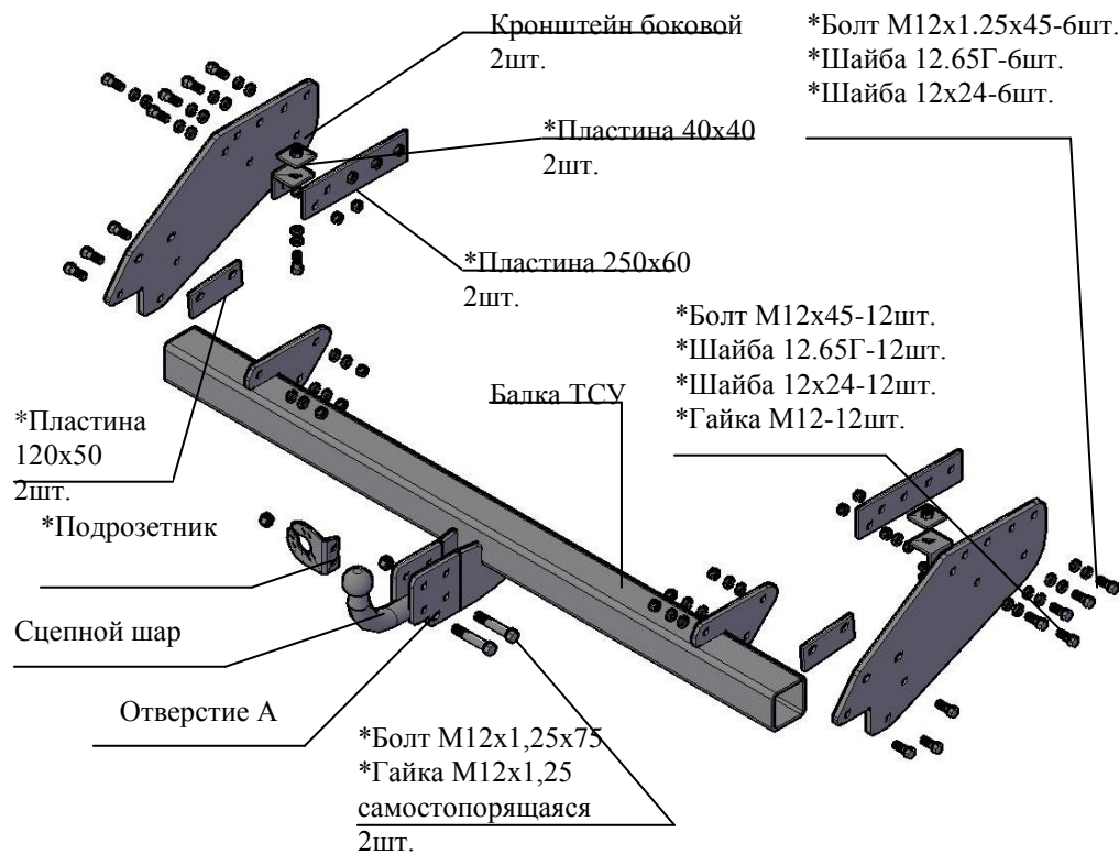
Рис.1 Тягово-сцепное устройство 7112
